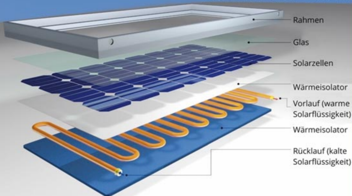
Abbildung 1: Aufbau eines PVT-Kollektors ( https://sonnenstrom365.de/was-ist-pvt/ )
